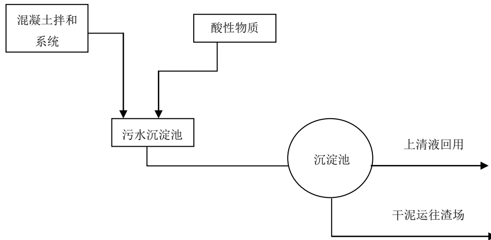
图 6.1-1 混凝土拌和系统废水处理工艺流程图
